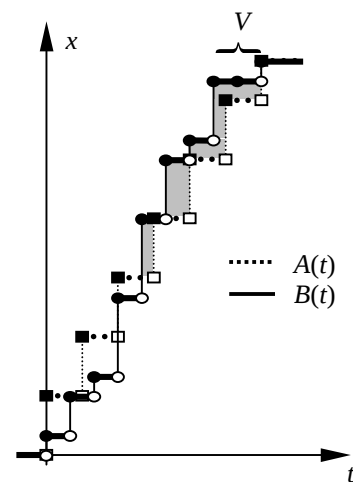
Bild 2c Vorlauf V
